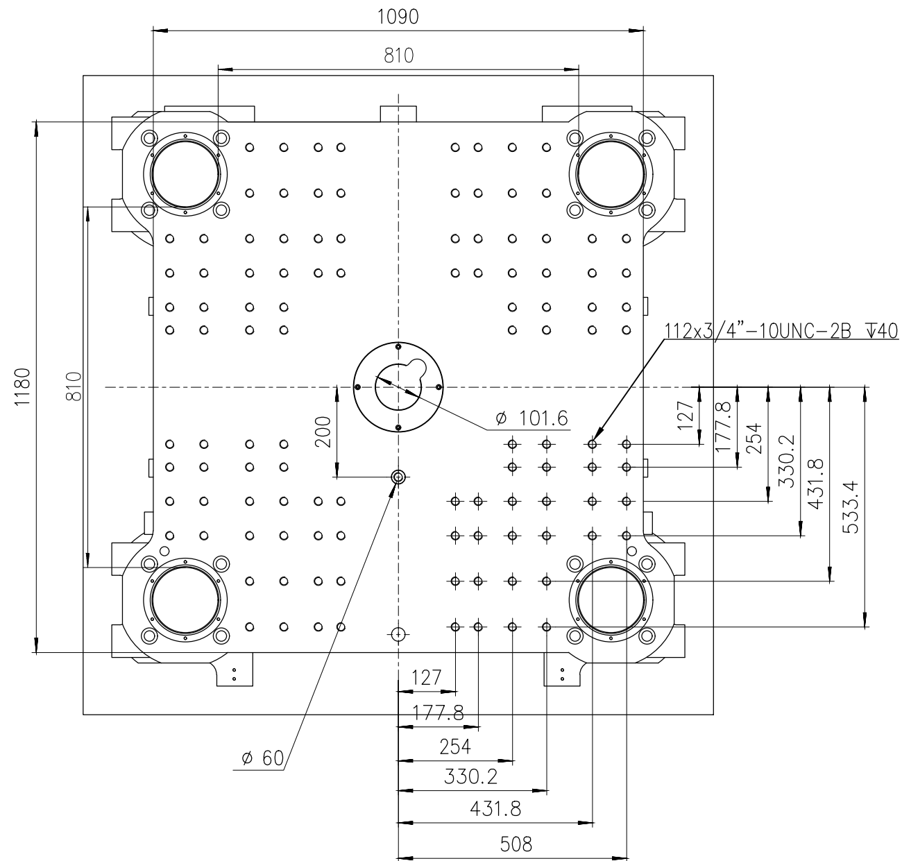
Fixed Platen
